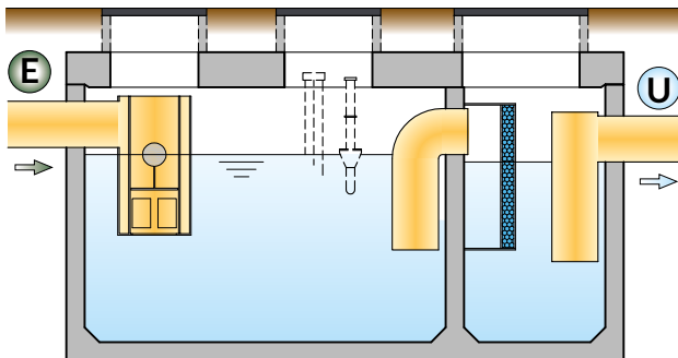
SEZIONE
